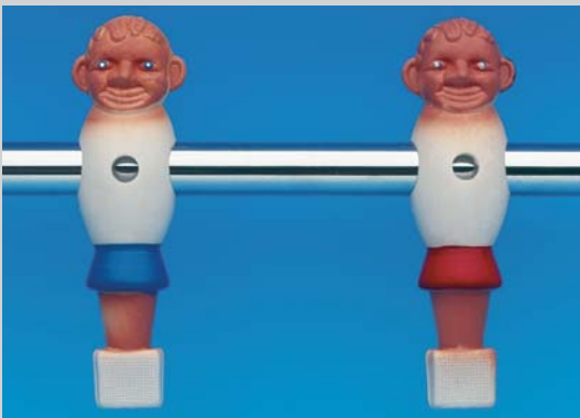
193.2014 Plastikfigur Economy blau 16 mm 193.2015 Plastikfigur Economy rot 16 mm Schraube: 191.1018 Mutter: 191.1006
